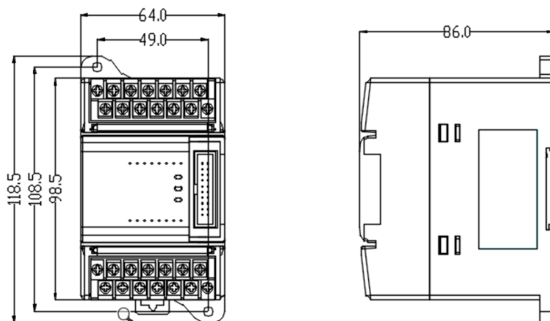
图 11-1 SCU系列扩展模块外观尺寸
