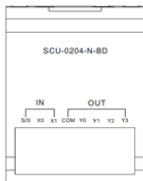
图 10-2 SCU-0204-N-BD模块端子丝印
