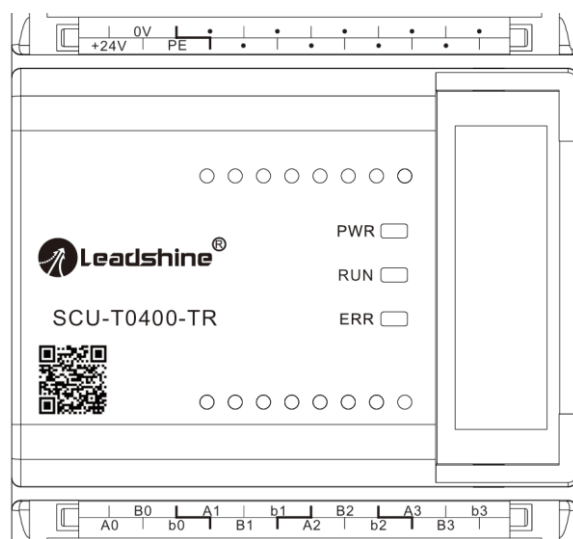
图 8-2 SCU- T0400-TR模块端子丝印
