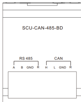
图 12-2 SCU-CAN-485-BD模块端子丝印
