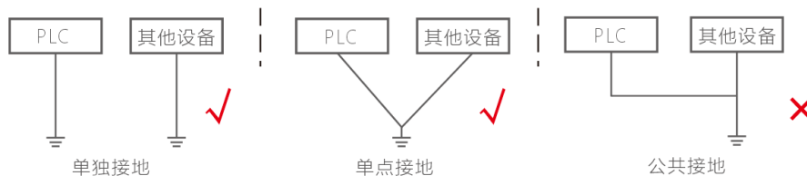
图 1-1 接地类型图
